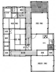
1階平面図 1/100
