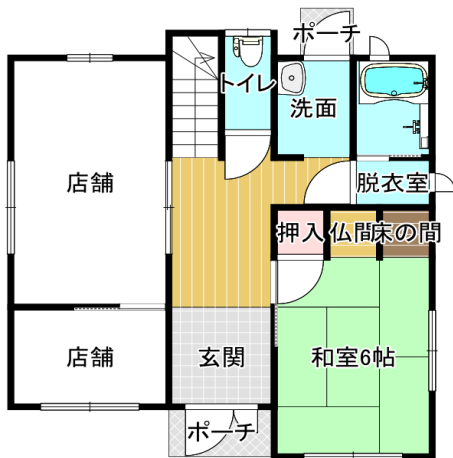
1階平面図
